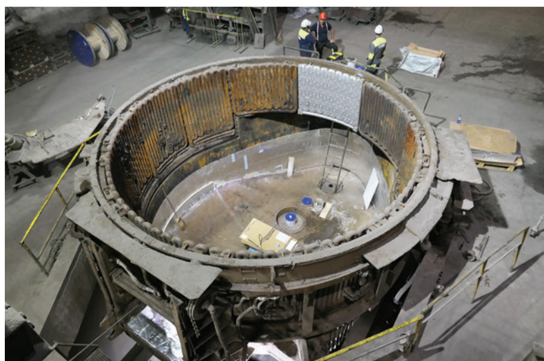
Oprava nístej EAF po demontáži výmurovky.
