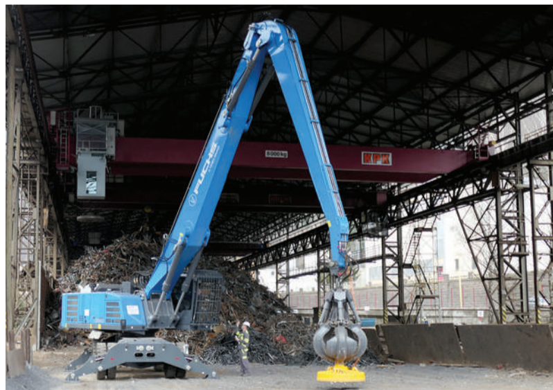
Nový mobilný manipulátor FUCHS je využívaný na homogenizačnom šrotovom poli v starom závode. Foto: M. Gončár
