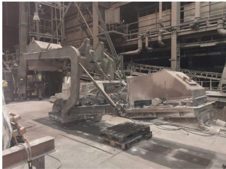
Pohľad na demontovaný otočný dopravník pece EAF, na ktorom sa uskutočnila výmena podvozkov a koľaje otoče. Foto: M. Oravec
