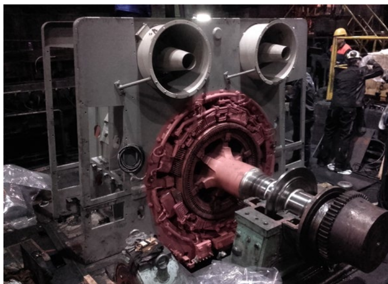
Výmena statora motora pretlačovacej stolice vo valcovni bezšvíkových rúr. Foto: I. Farárik
