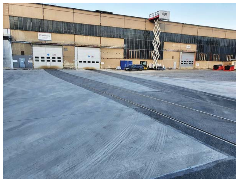
Odstavná plocha ťahárne rúr po realizácii opravy.
