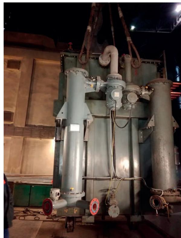
Výťahovanie starého transformátora EAF z trafokobky
