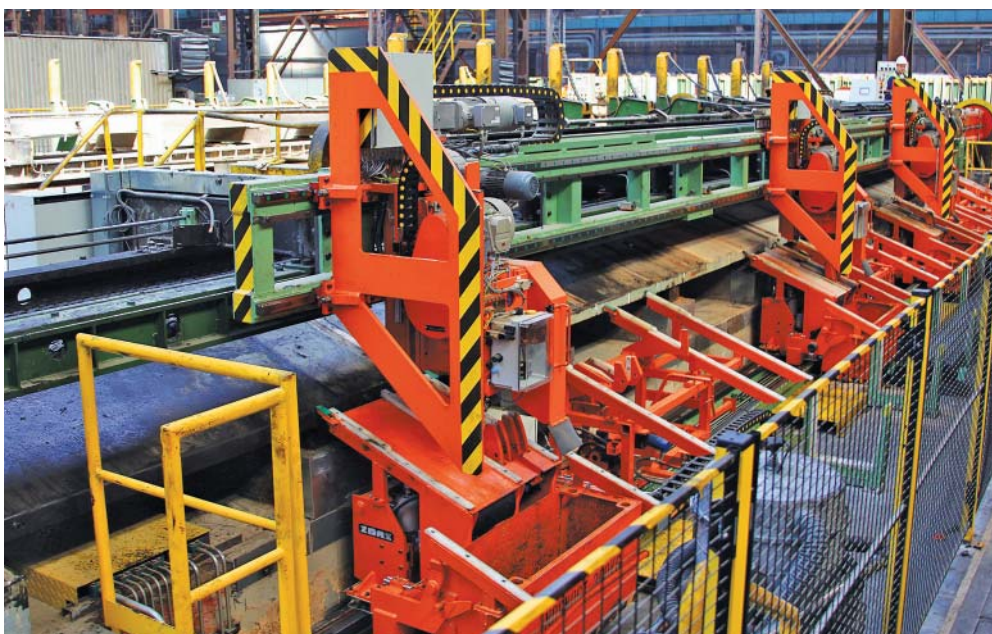
Medzioperačné delenie na ťahnej stolici 3-04.
