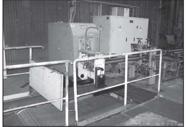
Nový indukčný ohrev pre výrobu oblúkov.
