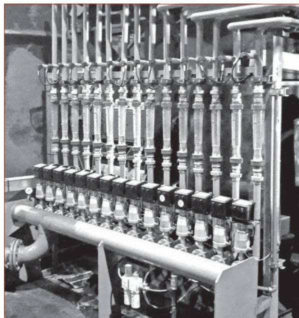
Regulačný stojan chladenia valcov redukovne
