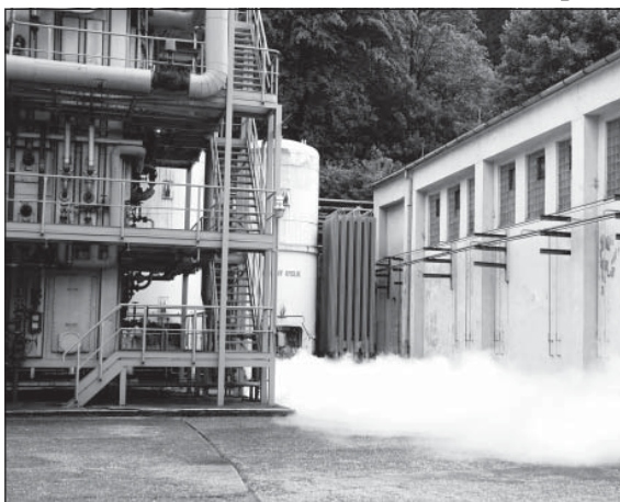
V priestoroch kyslíkárne bol simulovaný kontinuálny únik kvapalného kyslíka zo zásobníka FEROX na spevnenú plochu pod zásobník
