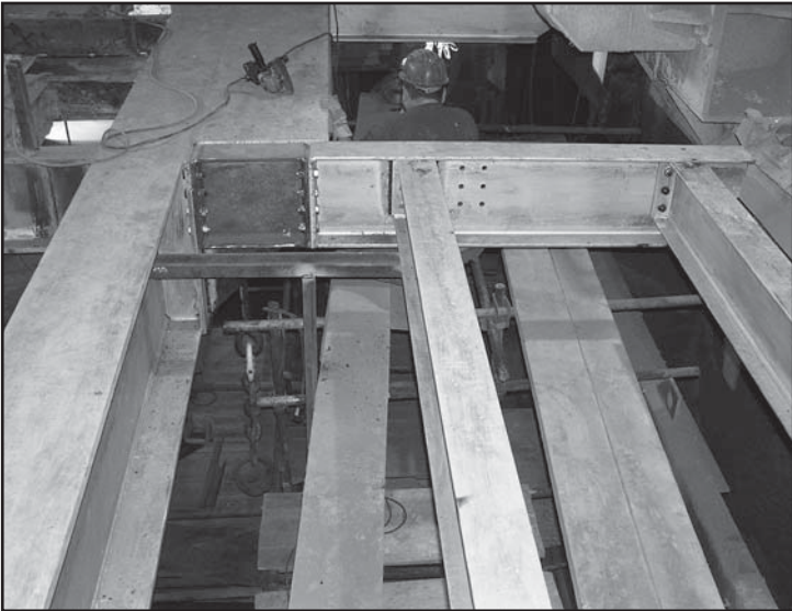
V prvej polovici júla bola v oceliarni zrealizovaná výmena nosníka 1 800 na plošine vo výške
