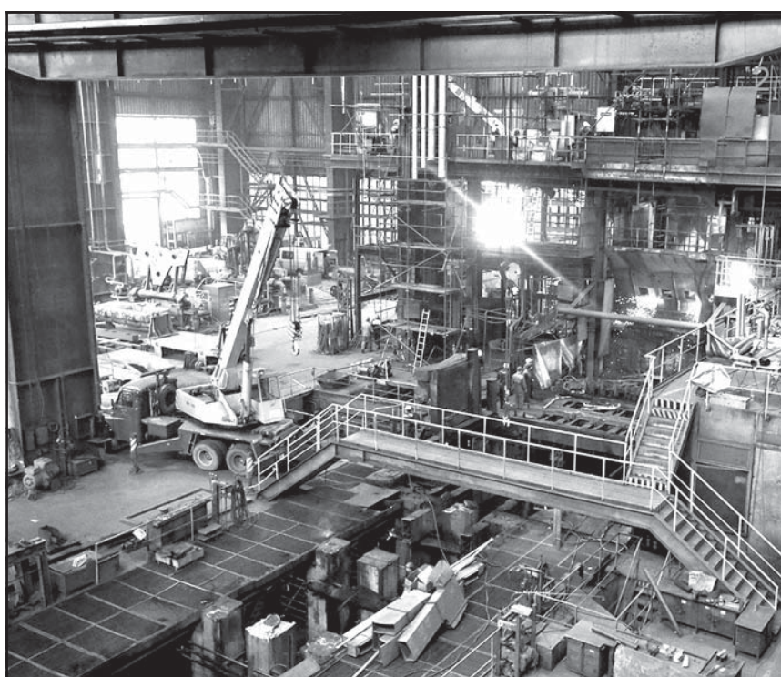
Demontážne práce starého zariadenia plynulého odlievania ocele počas druhého dňa odstávky – 2. septembra 2013 ráno
