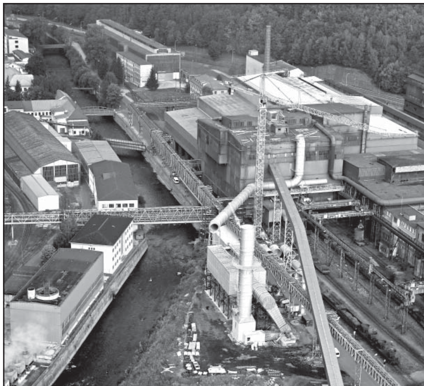
Posledný deň prevádzky oceliarne pred rekonštrukciou odprášenja elektrických pecí – 31. august 2013
