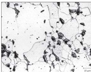
Obr. 10 priečný rez
