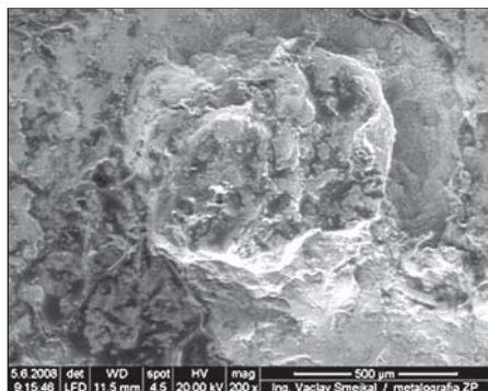
Obr. 4 „tuberkula“
