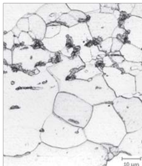
Obr. 9 pozdĺžny rez
