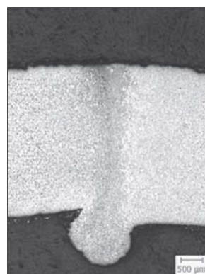
Obr. 6 priečný rez
