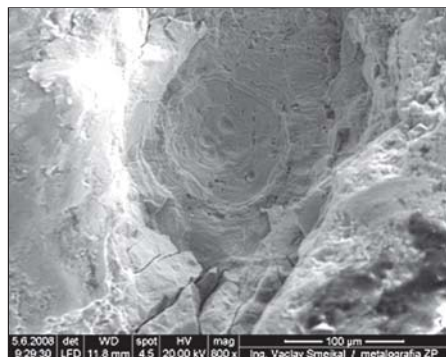
Obr. 5 korózna jamka
