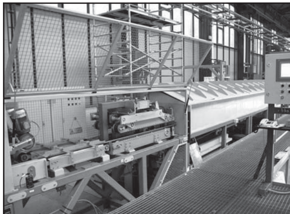
Najvýznamnejšou a zároveň najzložitejšou technologickou investíciou bola realizácia špeciálnej kontinuálnej dvojžilovej galvanickej linky na pozinkovanie HPL rúr. F: A. Nociarová
