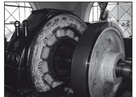
Generátor G2 po demontáži vonkajších krytov
